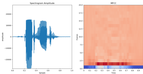
Gambar 11. Fitur MFCC Perintah Corner (Arif)
