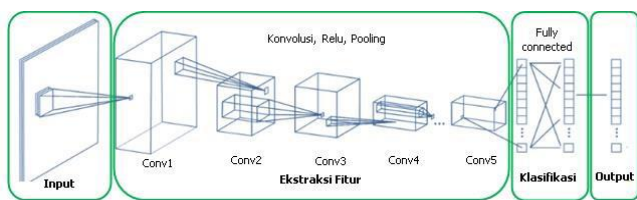
Gambar 5. Arsitektur CNN [7]
