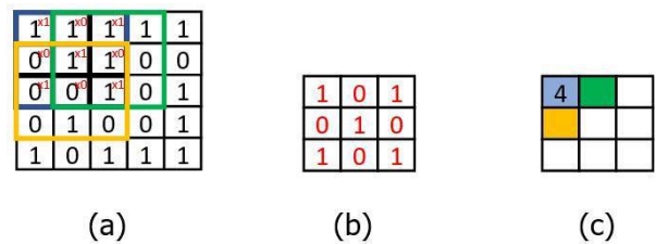
Gambar 6. Proses Konvolusi [7]
